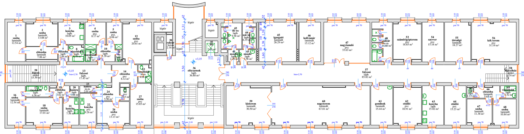
Móra Kollégium Közép fasor földszint alaprajz
