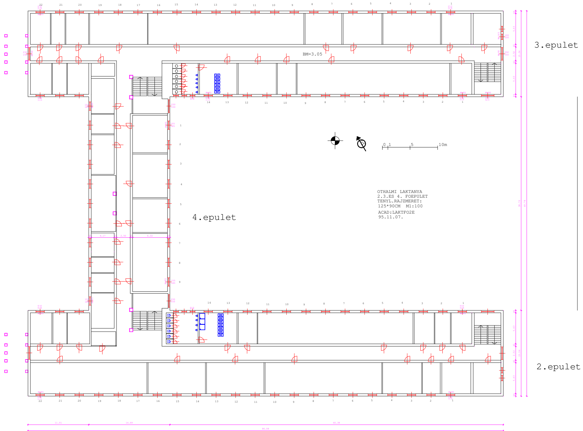
2.EMELET ALAPRAJZ
