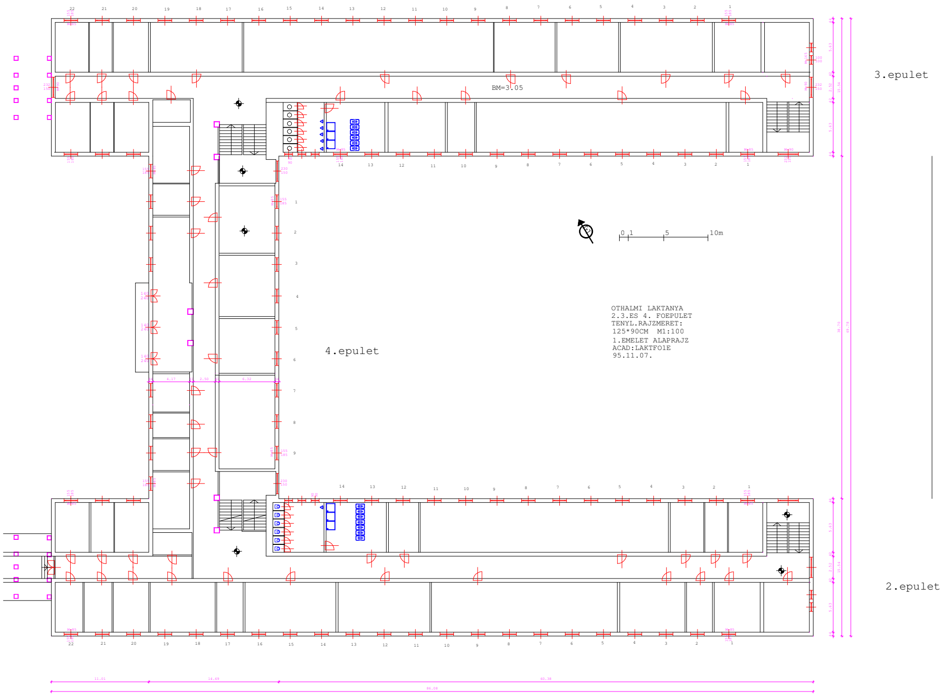
1.EMELET ALAPRAJZ
