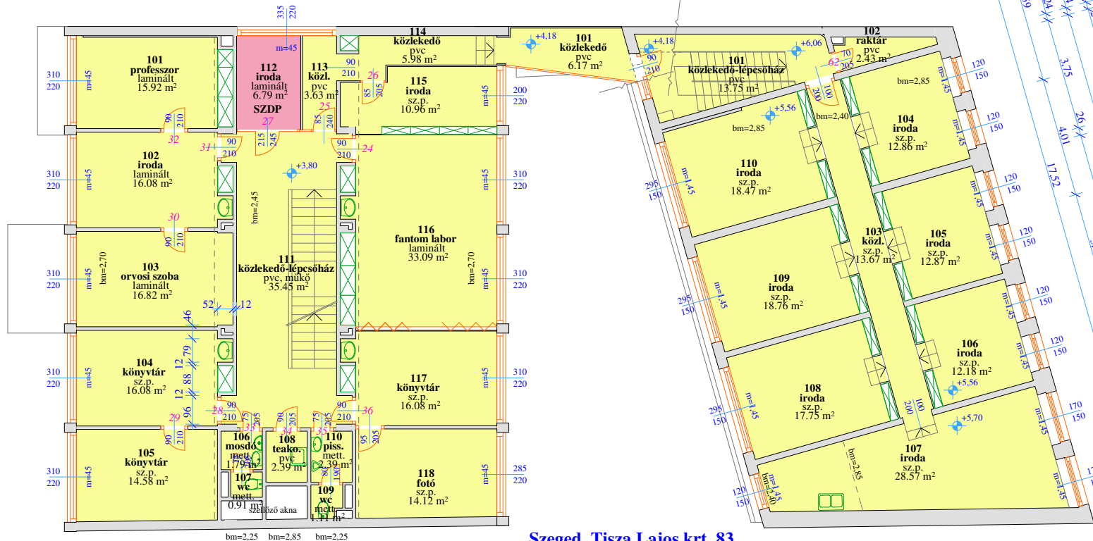
Szeged, Tisza Lajos krt. 83. 1.emelet alaprajz 2012.december
